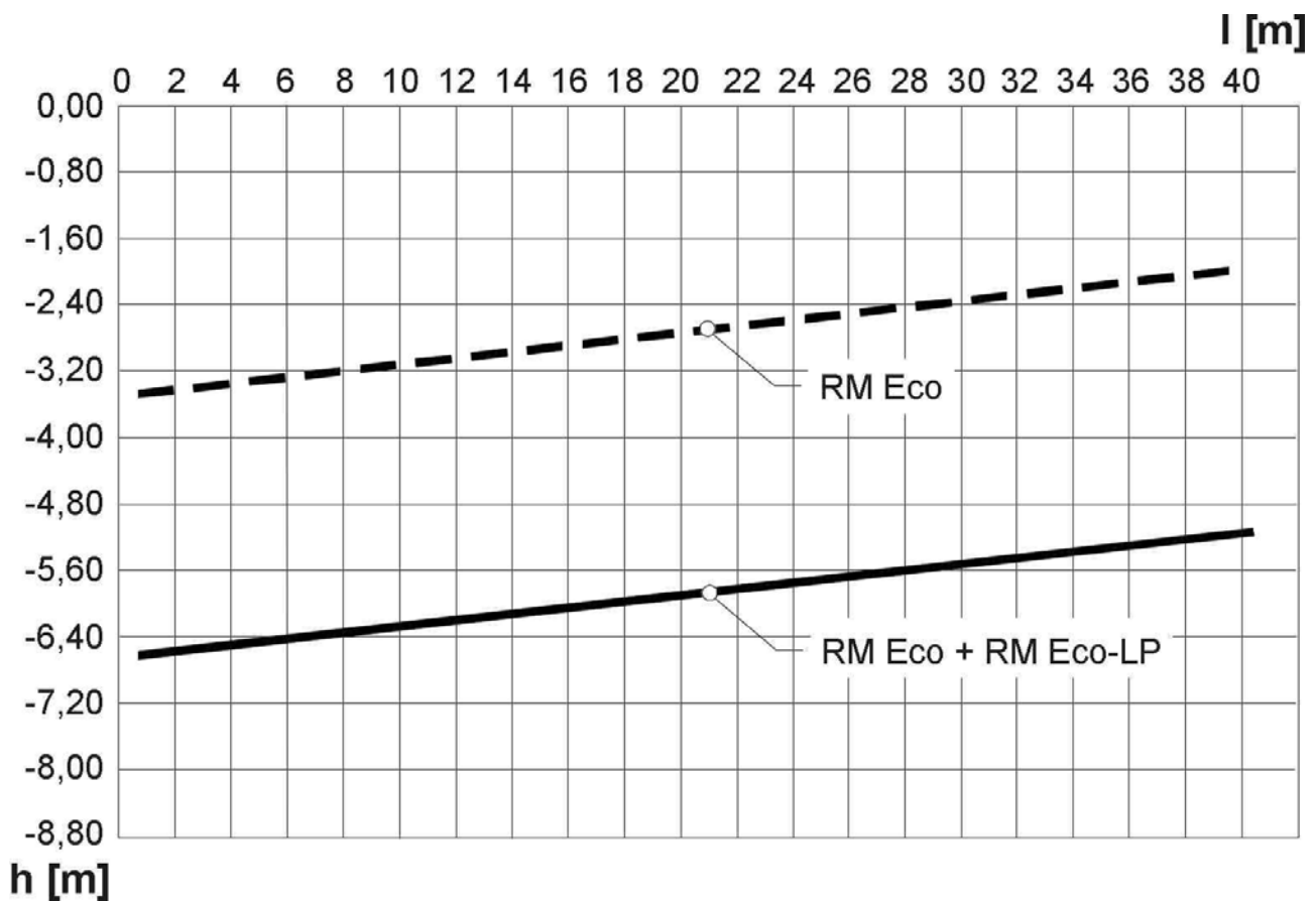
Ansaugkennlinie mit und ohne Ladepumpe RM Eco-LP .
