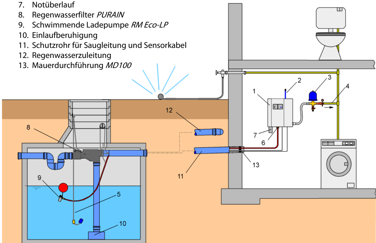
Beispielübersicht einer Regenwassernutzungsanlage mit RM Eco und Ladepumpe RMECO-LP im Speicher
